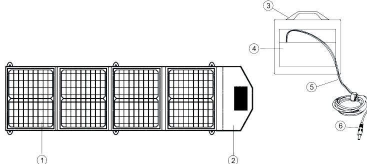
Obrázek č.1 – Technický popis solárního panelu VIKING L50
