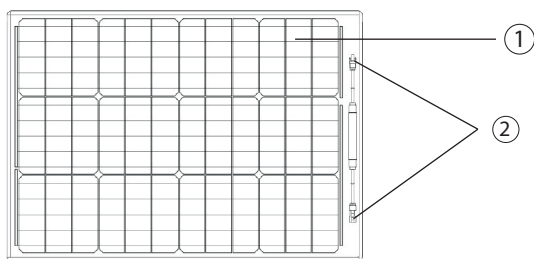
4. ábra - A VIKING LE60 és a VIKING LE100 napelem műszaki leírása
