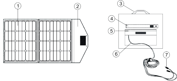
Obrázek č.2 – Technický popis solárního panelu VIKING L80 a L110
