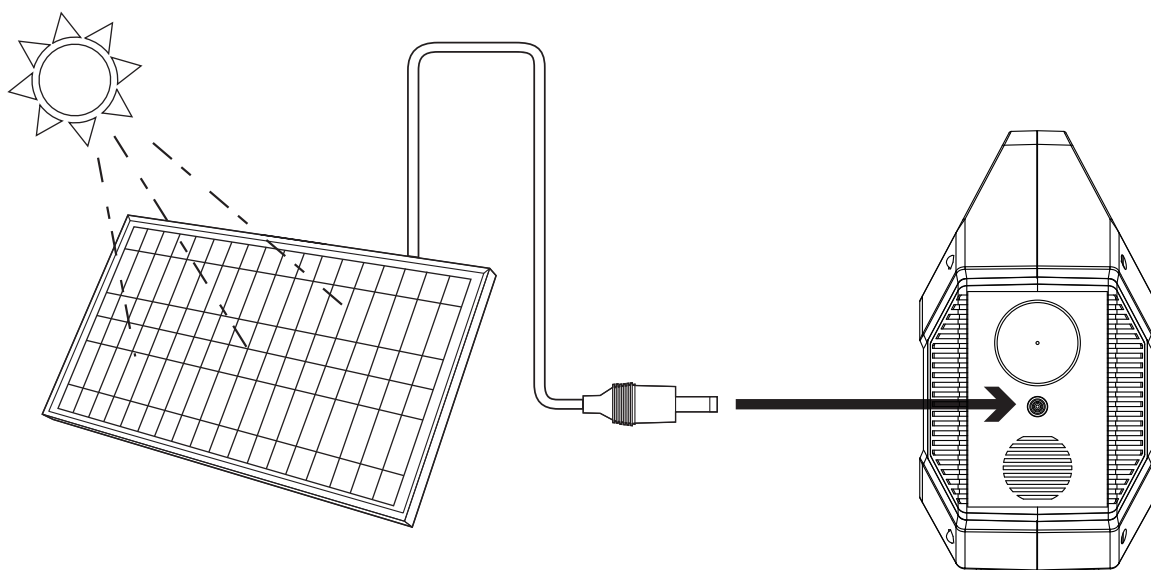
Solar Panel - výstup MPPT 13~25V, 2.1A Max
